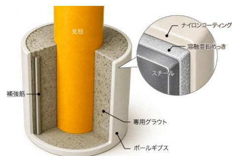
ポールギブスの断面構造イメージ
