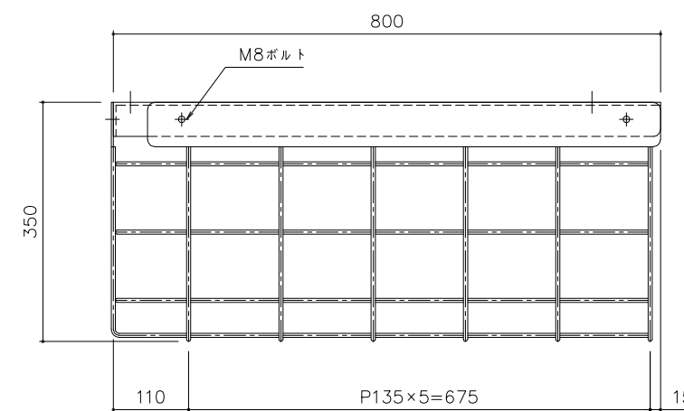
防球ガード(ツイストバー仕様) 材質: SS400・SPCC 概算重量: 18kg
