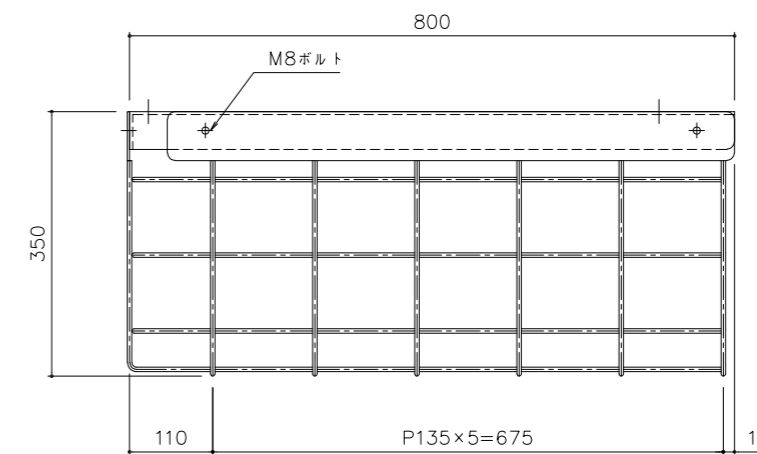
防球ガード(ツイストバー仕様) 材質: SS400・SPCC 概算重量: 23kg
