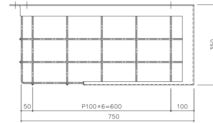
防球ガード(ツイストバー仕様) 材質: SS400・SPCC 概算重量: 30kg
