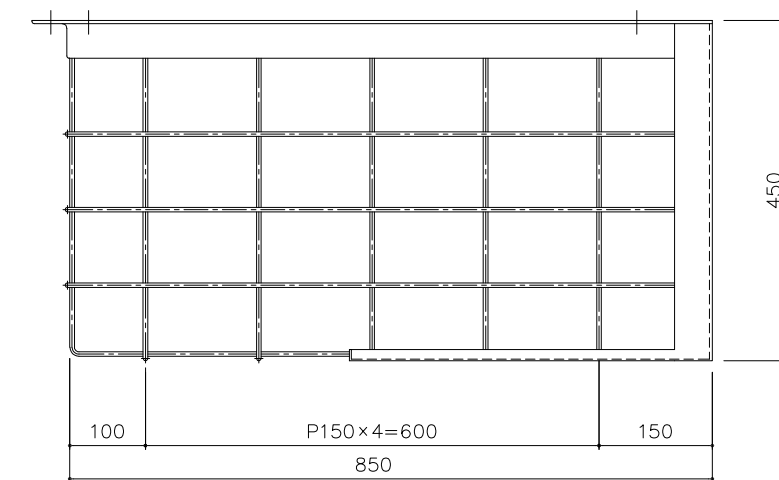
防球ガード(ツイストバー仕様) 材質: SS400・SPCC 概算重量: 33kg
