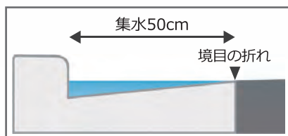
L型街渠
